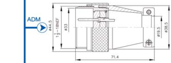
PLS-35-ADM
